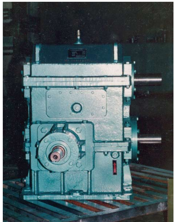
Redutor especial de eixos ortogonais e duplo eixo de saída
