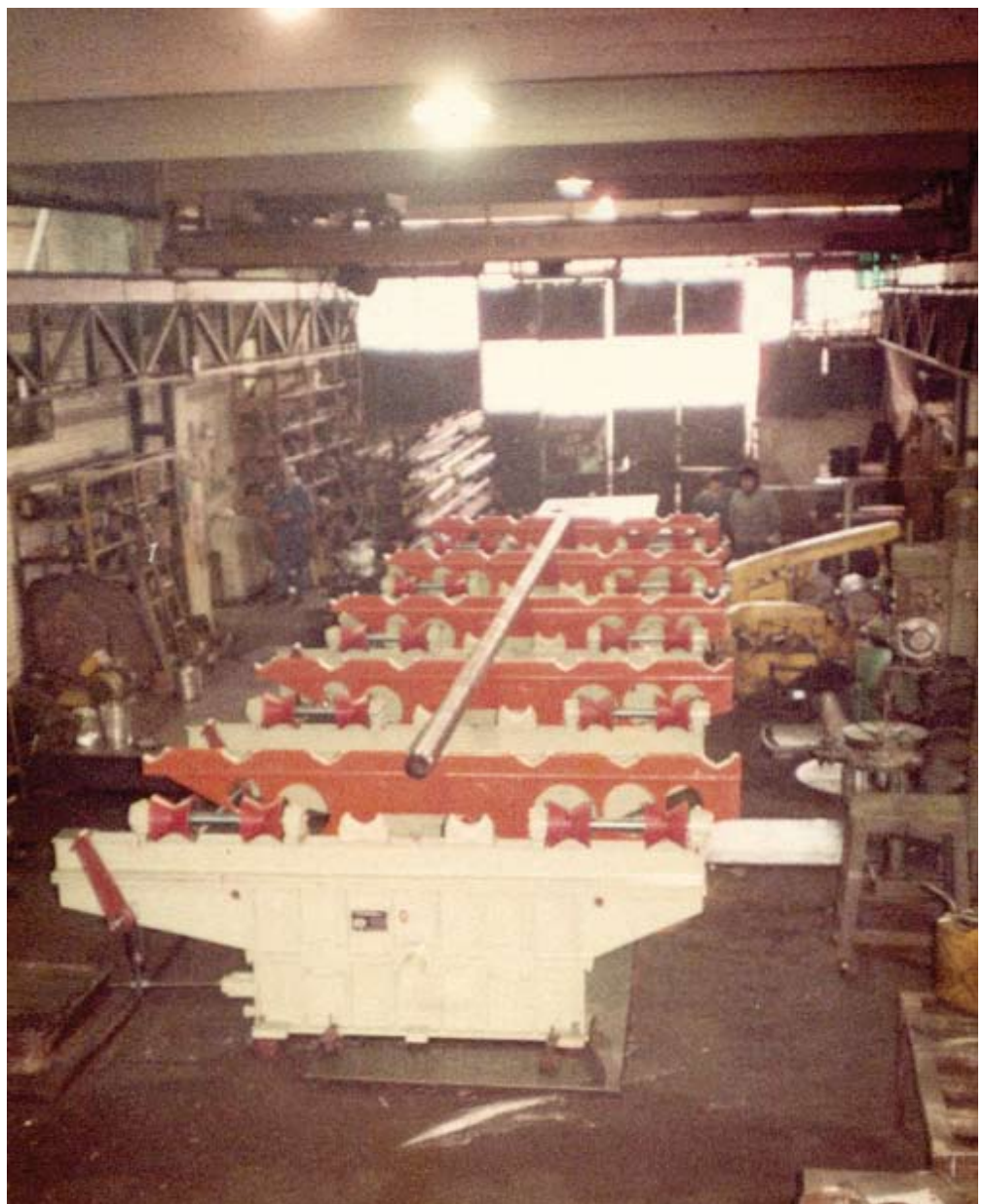
Transferidor de tubos fabricado para Siderca del grupo Techint
